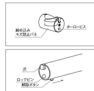
フェイスアーム 又はハンガーバー
