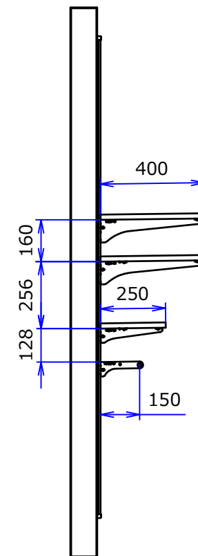
A-A ( 1 : 20 )
