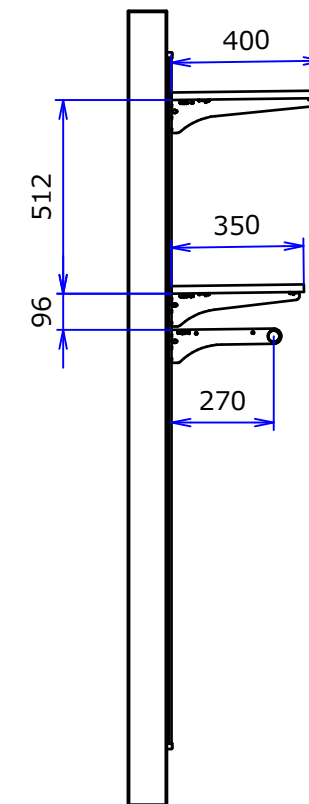
B-B ( 1 : 20 )
