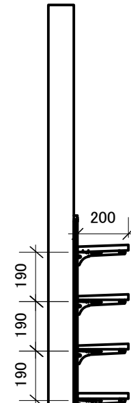
A-A ( 1 : 20 )
