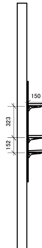
B-B ( 1 : 20 )
