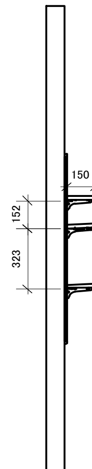
A-A ( 1 : 20 )
