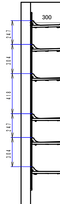
B-B ( 1 : 20 )
