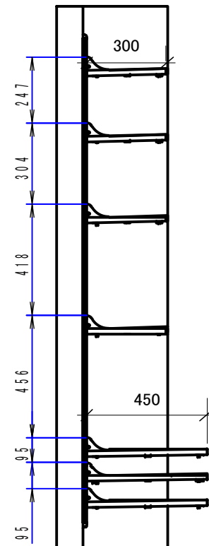
A-A ( 1 : 20 )
