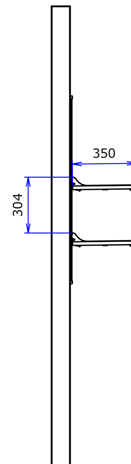
B-B ( 1 : 20 )
