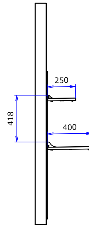
A-A ( 1 : 20 )
