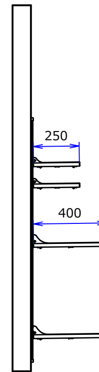
B-B ( 1 : 20 )
