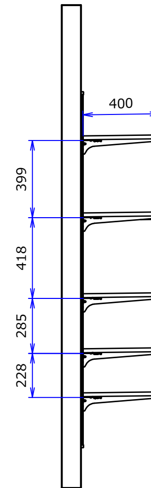
B-B ( 1 : 20 )
