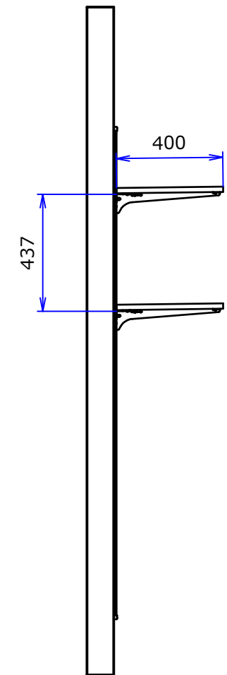
C-C ( 1 : 20 )
