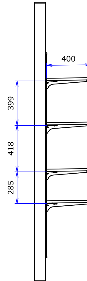
A-A ( 1 : 20 )
