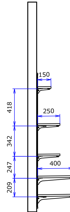
B-B ( 1 : 20 )
