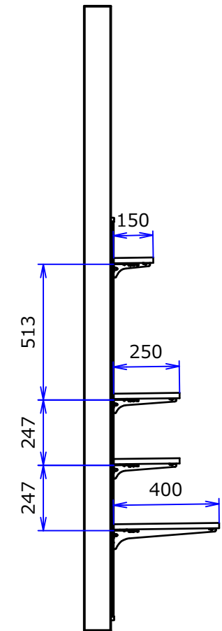
C-C ( 1 : 20 )
