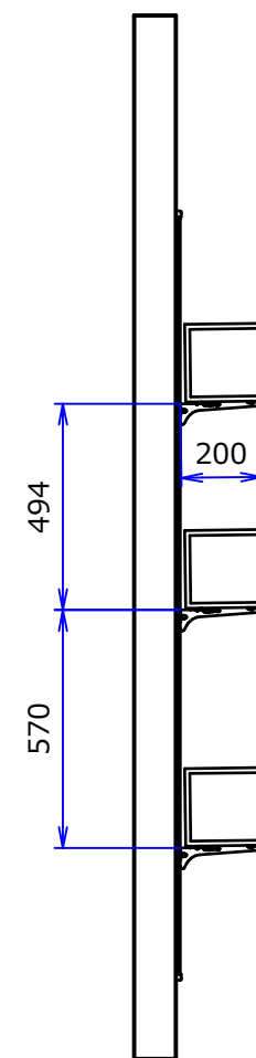
C-C ( 1 : 20 )
