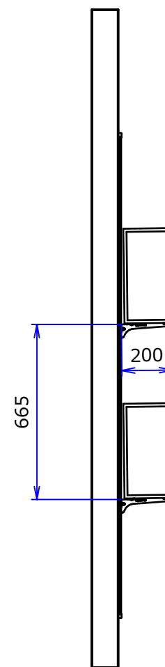
B-B ( 1 : 20 )
