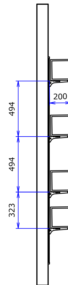
D-D ( 1 : 20 )
