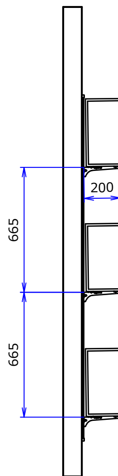
A-A ( 1 : 20 )
