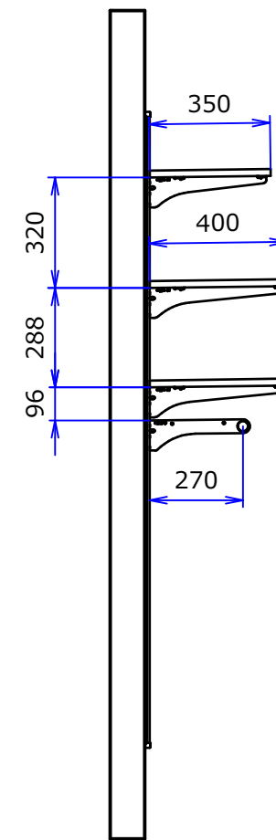
A-A ( 1 : 20 )
