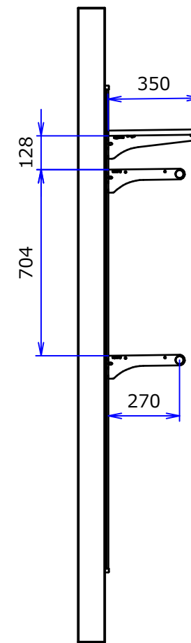
B-B ( 1 : 20 )
