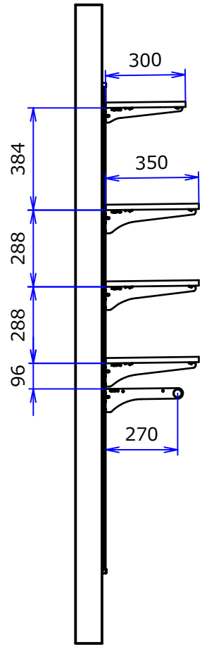
A-A ( 1 : 20 )
