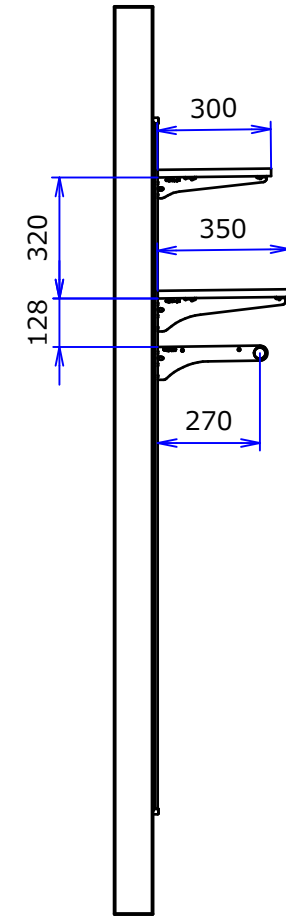
B-B ( 1 : 20 )
