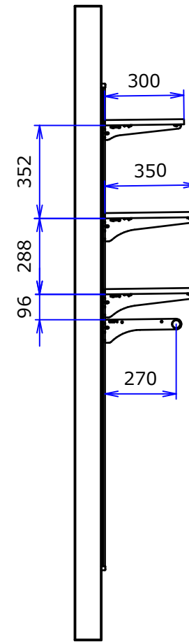
B-B ( 1 : 20 )
