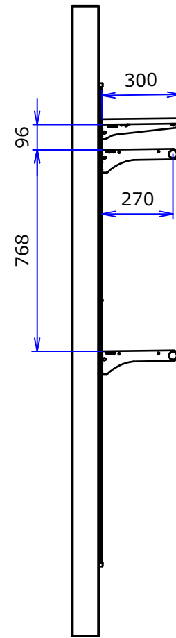
A-A ( 1 : 20 )
