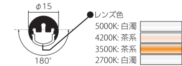
〈灯具断面図〉
